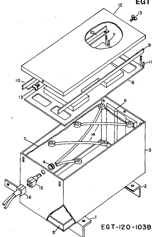
POWER PACK BOOSTER FOR EGT 120 - 150 EGT 200
